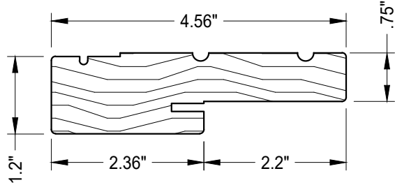
2 WOOD JAMB
